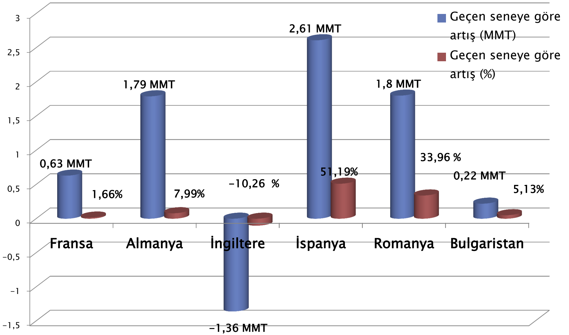
Grafik 1: Avrupa Birliği Ülkelerinin 2012 hasat yılına göre buğday üretimi artış miktarları ve yüzdeleri
